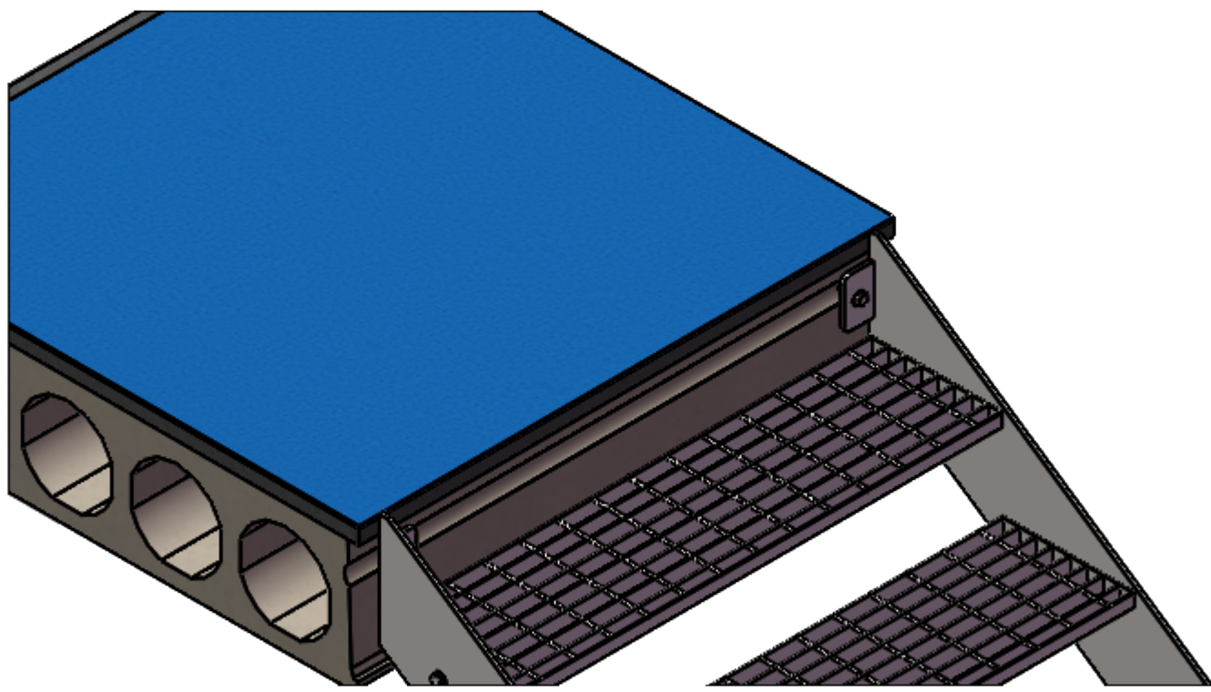
Infästning i HDF 90°.
