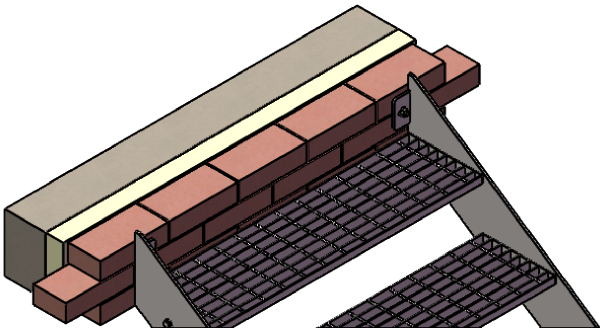
Infästning i tegelvägg.
