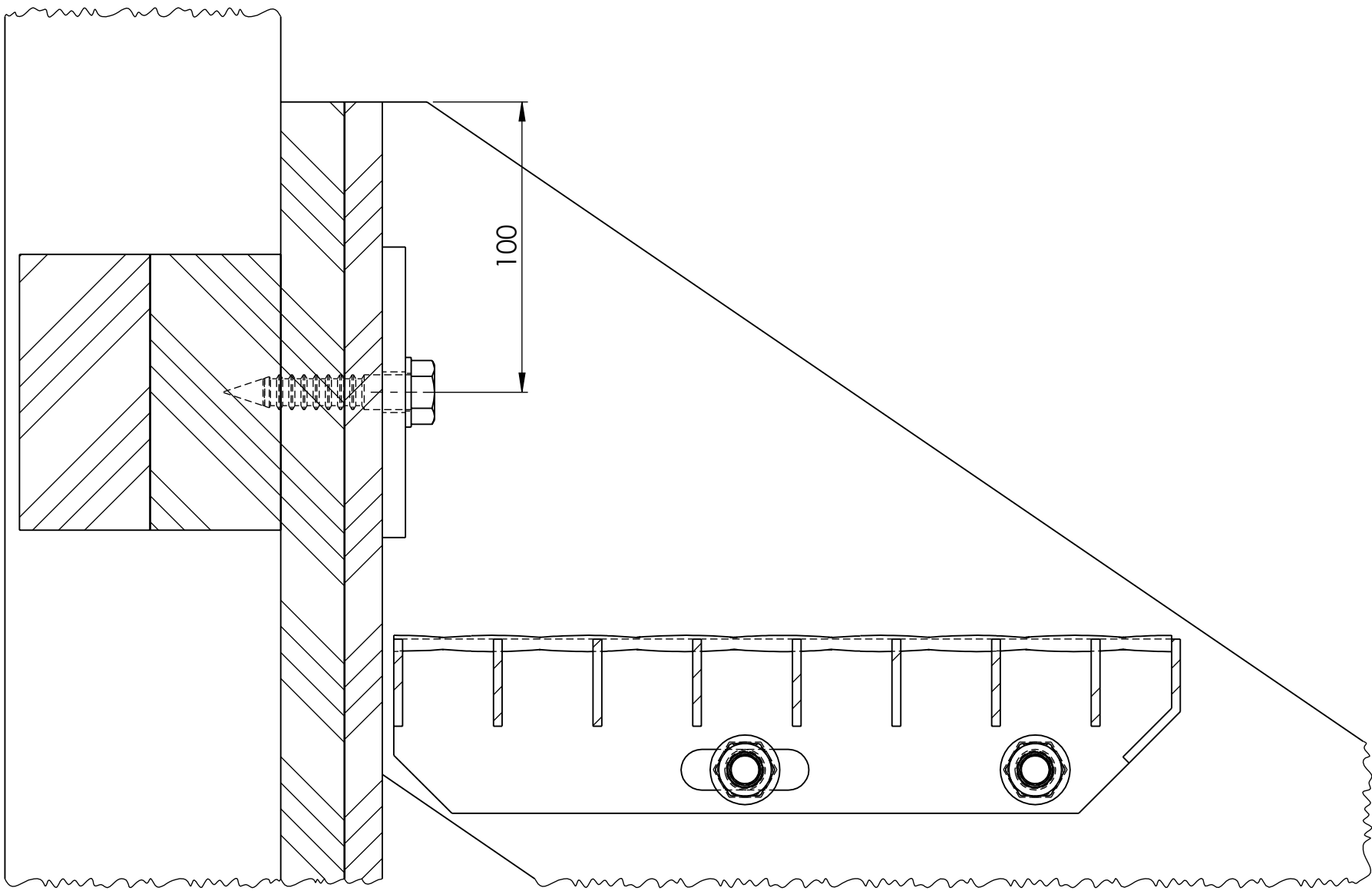
SECTION N-N SCALE 1 : 2
