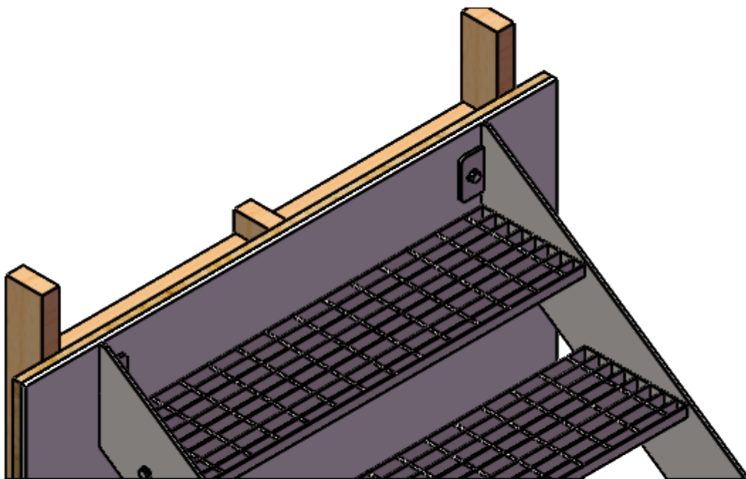
Infästning i regelvägg/OSB/Gips.
