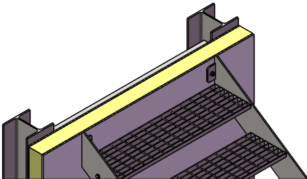
Infästning i sandwichpanel.
